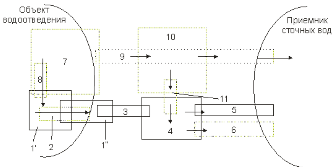
Рисунок 6 - Блок-схема водоотведения:
