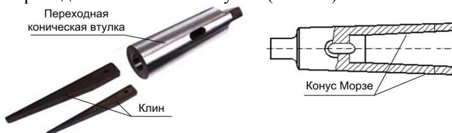
Рис.23 Переходные конические втулки и клин для извлечения инструмента
