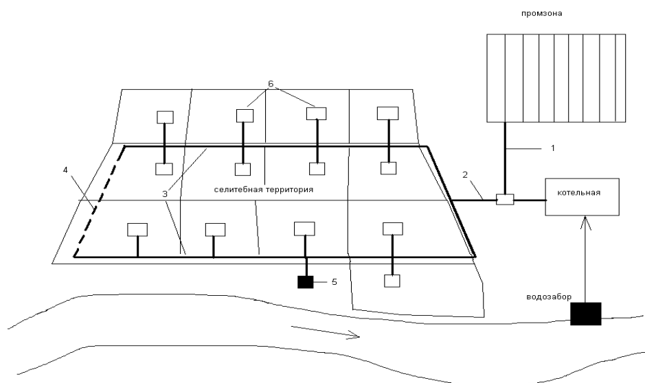
Рис.7. Схема централизованного теплоснабжения населенного пункта.
